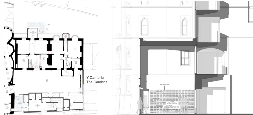
Cynllun Mynedfa i'r Atrium | Atrium Entrance Plan
